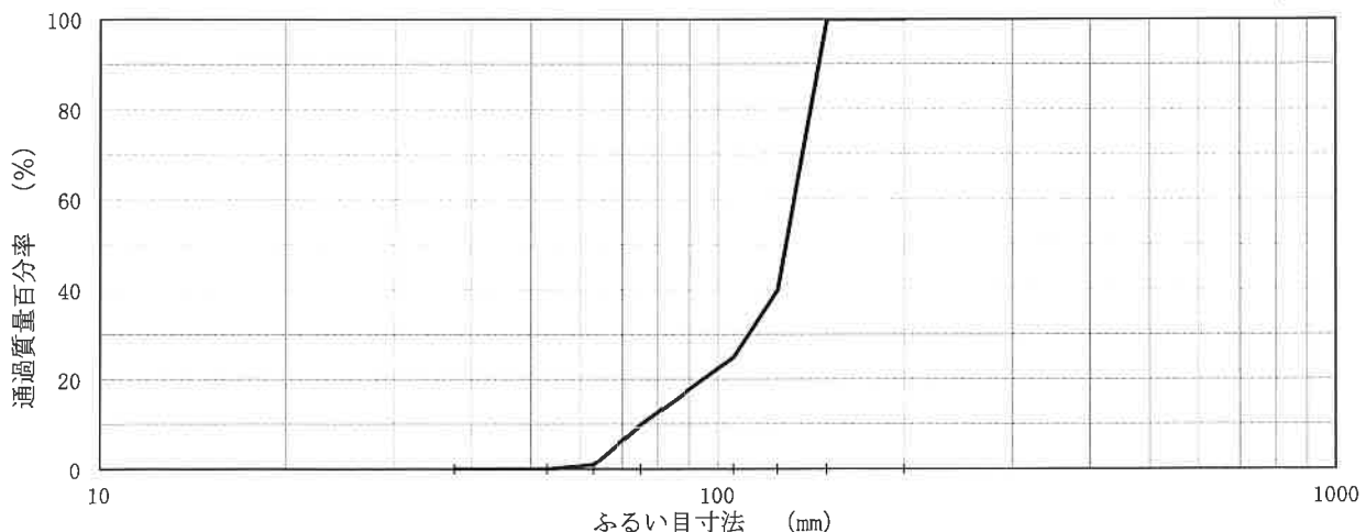
粒度分布曲線
